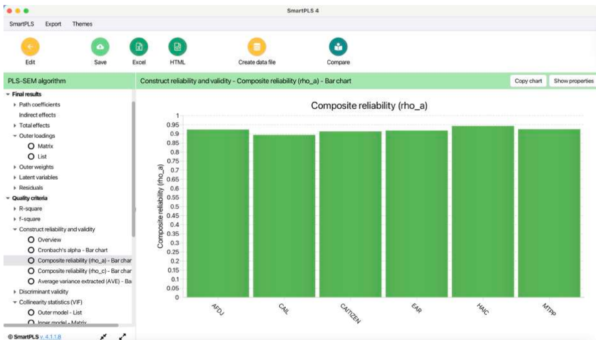
Figura 5.4. Gráfico de Composite Reliability rho_a .
